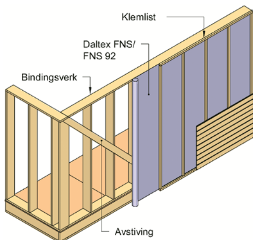
Fig. 2 Daltex FNS 92 / FNS 125 brukt som vindspærre på vegg.
